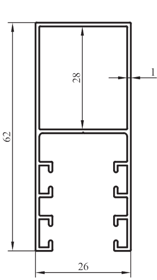
14172 0,580 kg/m
