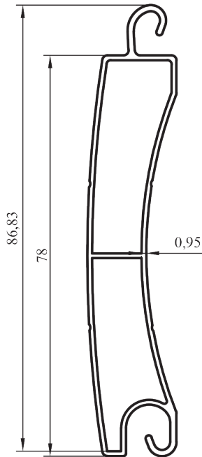
191221 0,602 kg/m
