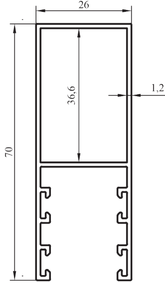
13025 0,720 kg/m
