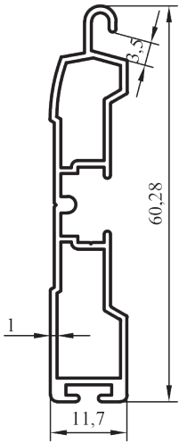
14426 0,440 kg/m
