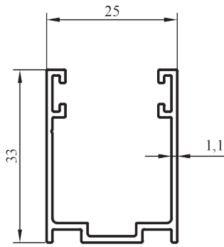
14256 0,330 kg/m
