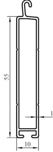
13022 0,380 kg/m
